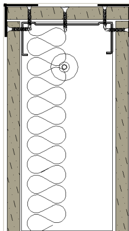
MUROS CABEZALES Y VANOS EN MUROS
