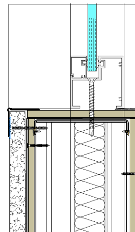
BORDES DE VENTANAS
